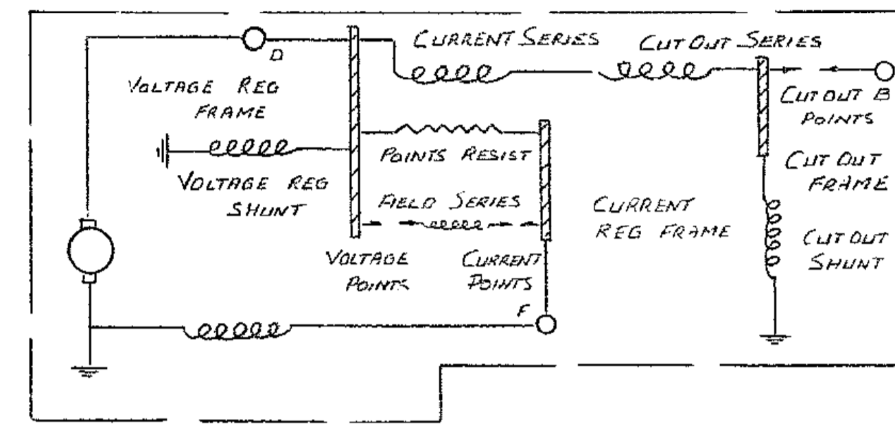
R.B. 310 CIRCUIT
